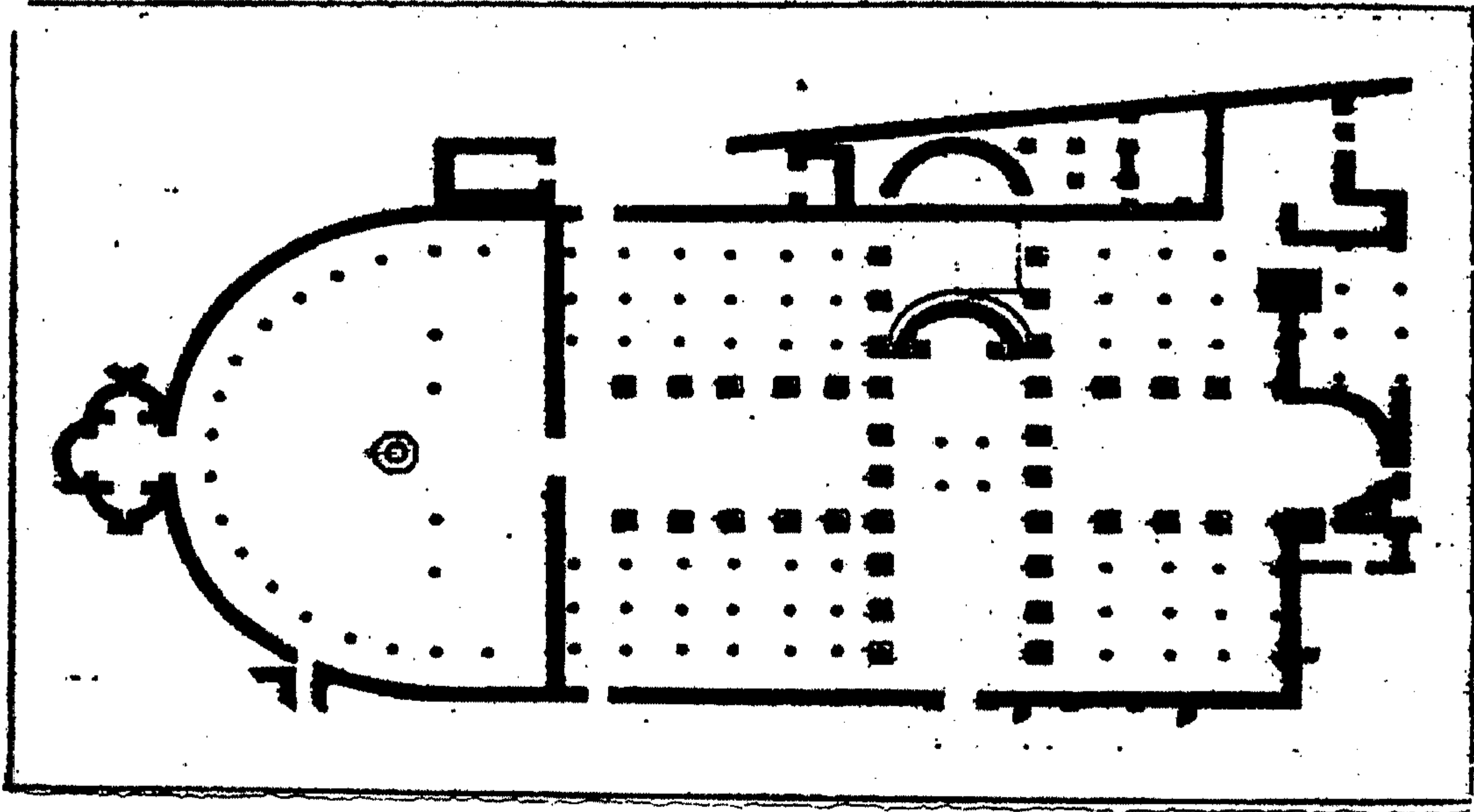
(شكل رقم ٣) رسم تخطيطي لكنيسة داموس الكاريتا عن د/ أحمد فكري
